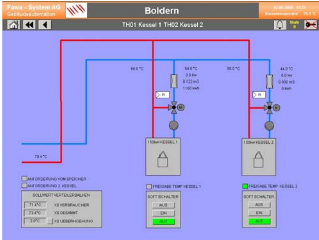
Webvisualisierung : Übersichtsbild Wärmeerzeugung Bedienung über Panel-PC in Wärmeverteilung oder beliebigem PC im Netzwerk
